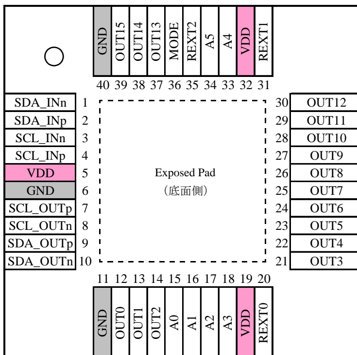
(上面図)
